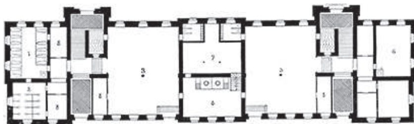
Fig. 472. — Plan du sous-sol, Echelle : 1/500. 1. Bains. — 2. Bouches. — 3 et 5. Salles de gymnastique. — 4. Chauffage central. — 6. Lingerie. 7. Combustible. — 8. Vestiaires.
