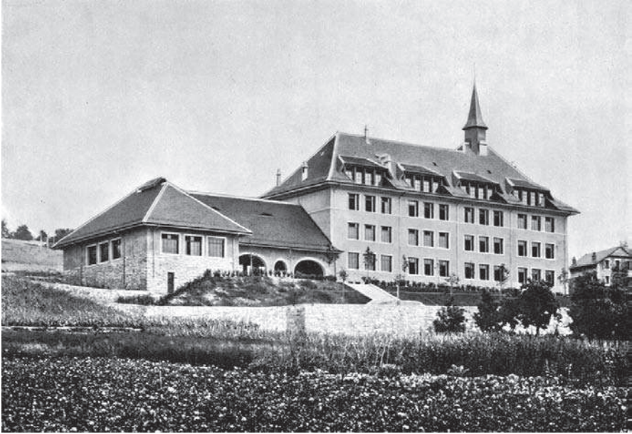
Fig. 8-11 : Pully (VD), à gauche, la salle de gymnastique et à droite, le bâtiment scolaire principal, reliés par un préau couvert.
